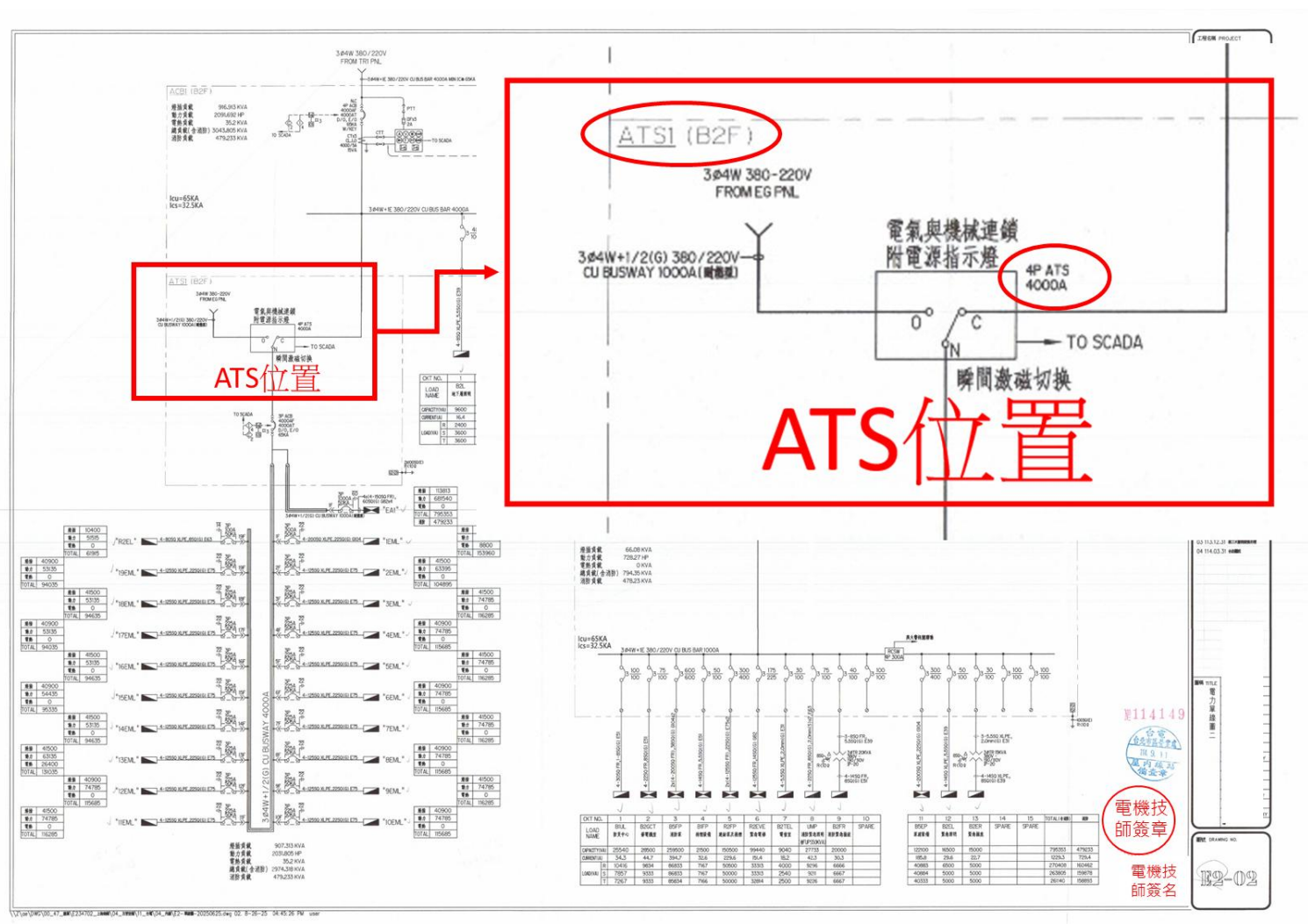
附件二、台電單線系統審迄圖(範例二)
