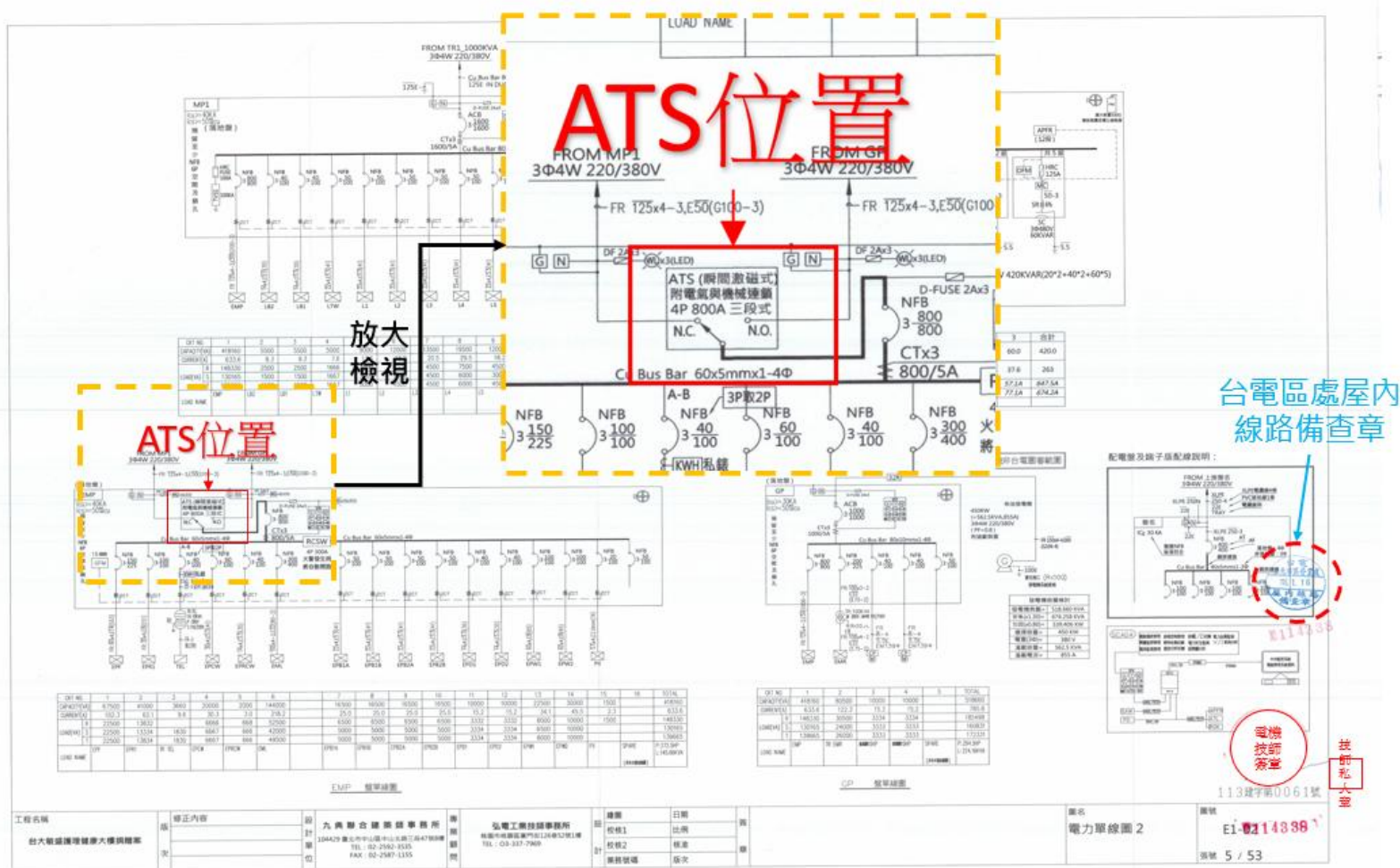
附件一、台電單線系統審迄圖(範例一)
